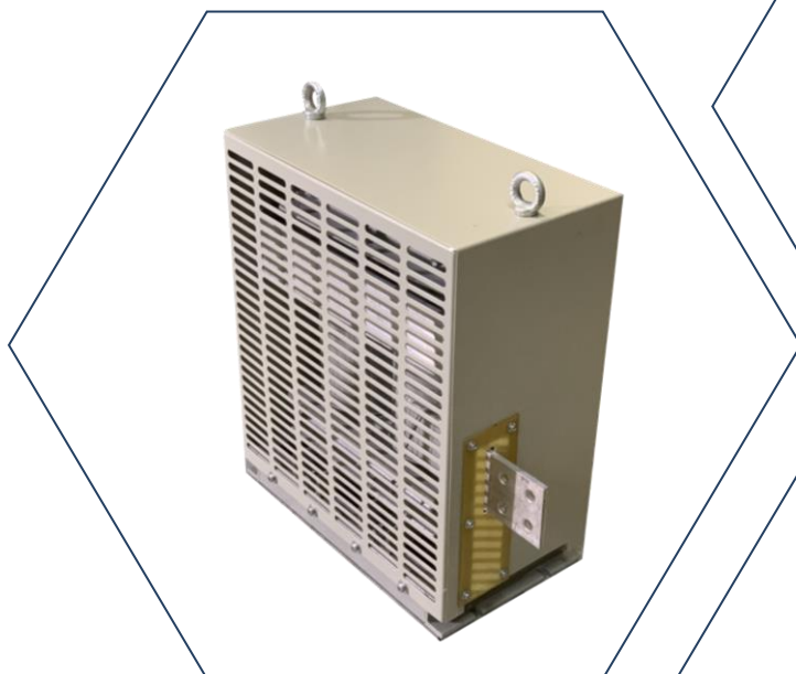
СГЛАЖИВАЮЩИЙ РЕАКТОР
